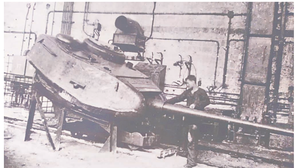
Сборка башни танка Т-44. Завод № 75 в Харькове.
