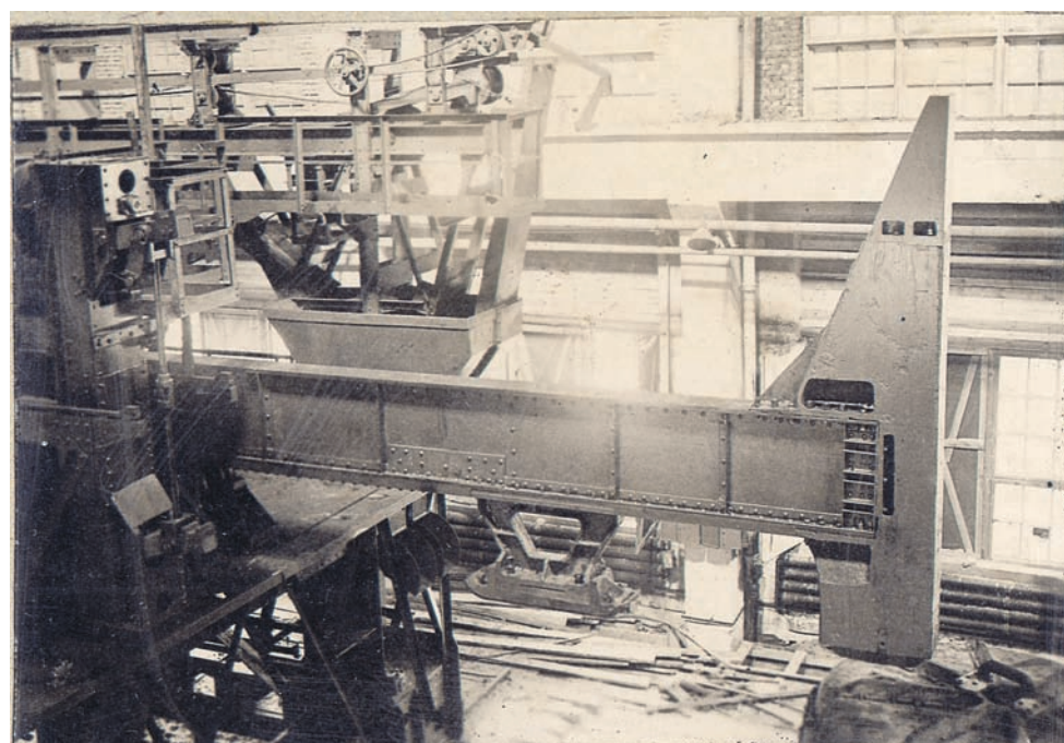
Монтаж выталкивающей штанги коксовыталкивателя на Коломенском заводе. Оригинал фотографии хранится в музее АО «Коломенский завод».
