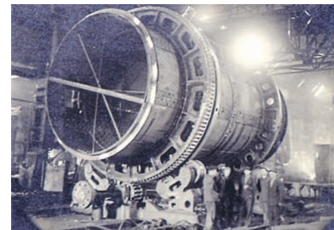
Монтаж конвертера на Коломенском машиностроительном заводе. Оригинал фотографии хранится в музее АО «Коломенский завод».
